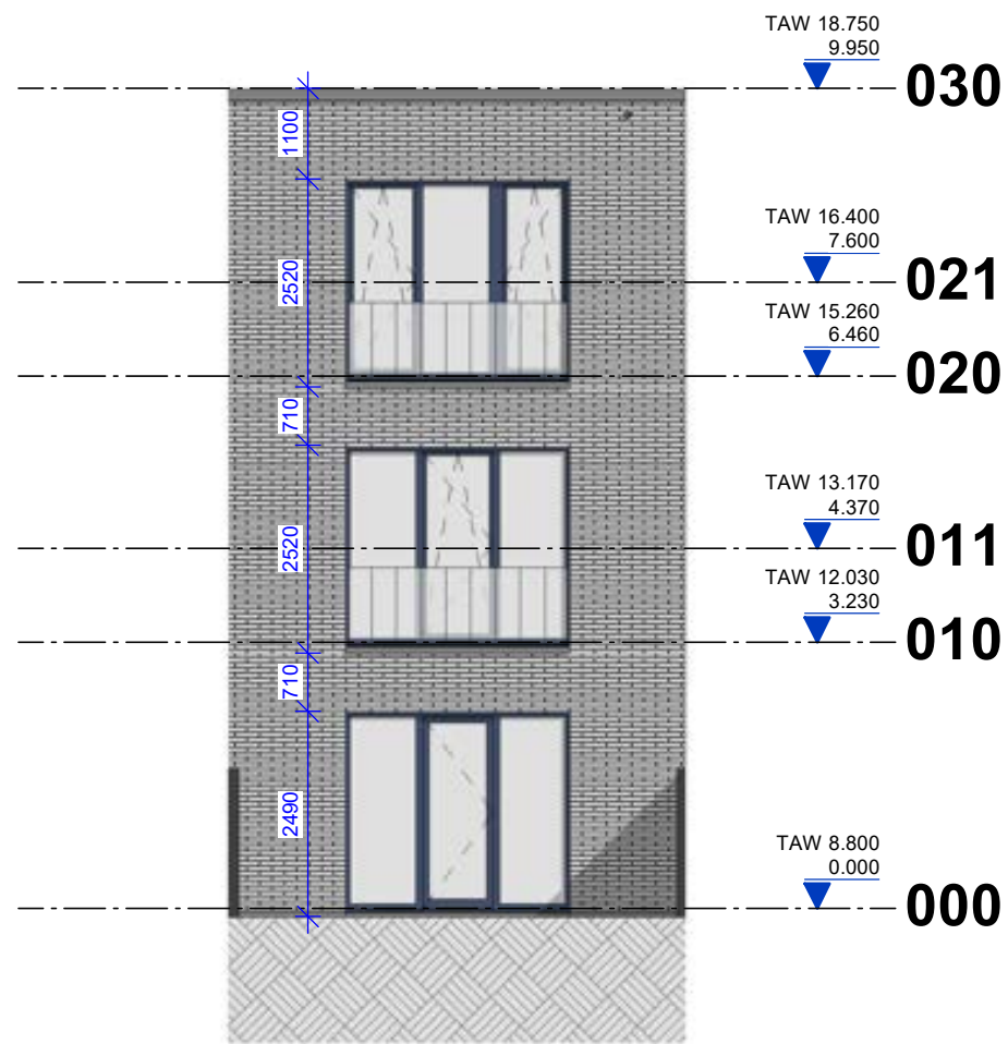
Schaal: 1 : 100 Achtergevel
