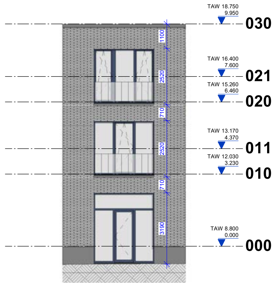
Schaal: 1 : 100 Voorgevel
